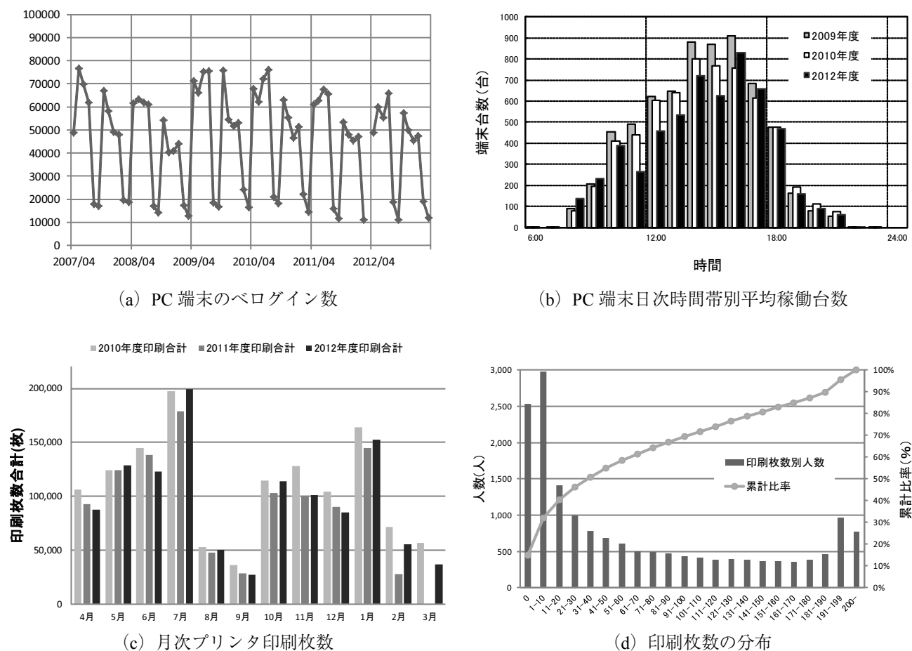
図 3.2.3：PC 端末およびプリンタ利用状況
