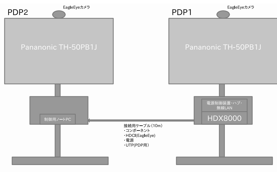
図 3.4.3：瀬戸内臨海実験所京都リサーチパーク遠隔講義システム概要図
